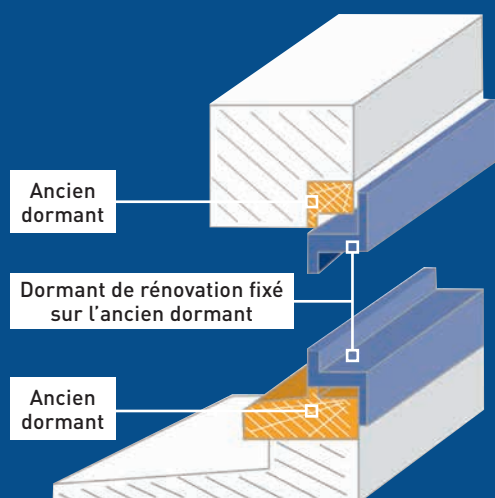
COUPE DE POSE EN RÉNOVATION
