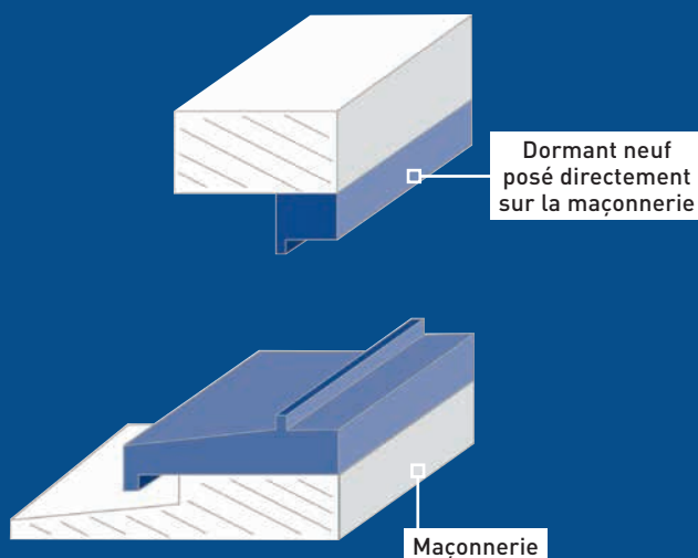
COUPE DE DÉPOSE TOTALE
