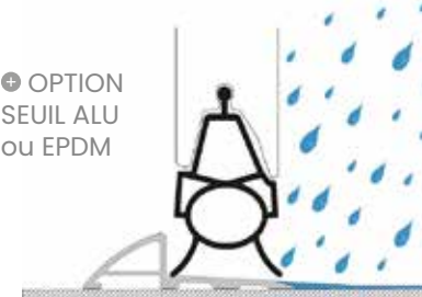
Joints périphériques ISO
